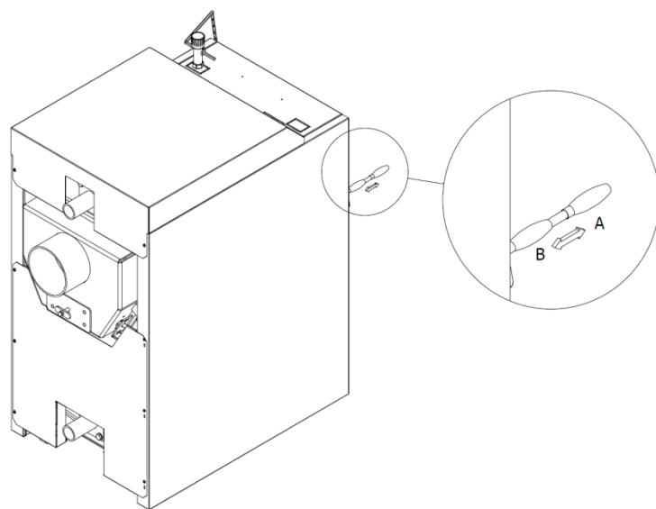
Obr. 21 Zátap v kotli W22 ECO
