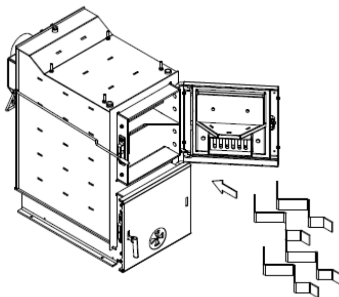
Obr.24 Umístění turbulátorů v kotli
